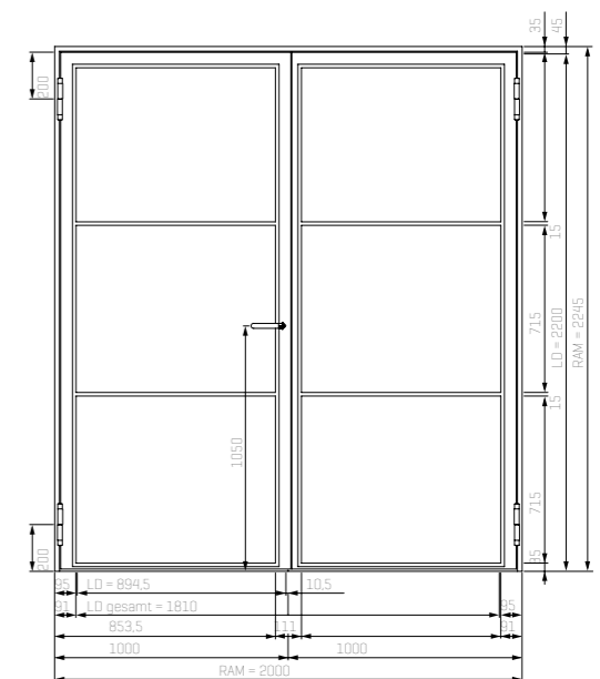
2-flüglige Stahl-Lofttür
