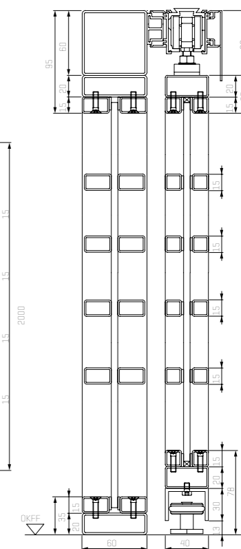
Vertikalschnitt 2-flüglige Stahl-Lofttür mit Seitenteilen
