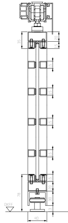
Vertikalschnitt 1-flüglige Stahl-Lofttür
